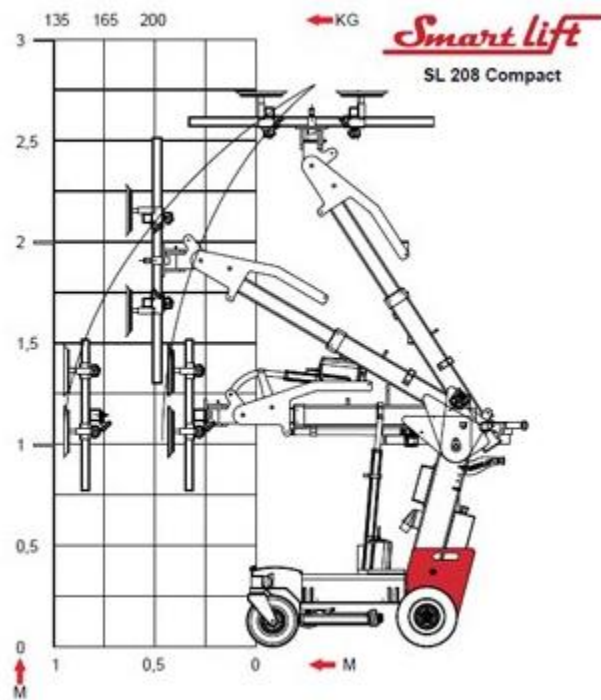
Διάγραμμα φορτίου ανύψωσης
